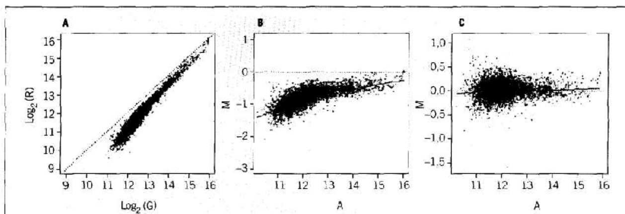
Fig. 6. Normalización de las intensidades del canal rojo (R) y verde (G) obtenidos en un experimento de reproducibilidad (la misma muestra marcada con diferente fluorocromo). A: gráfica \log(R) frente a \log(G) , donde se aprecia menor señal en la muestra marcada con el fluorocromo rojo. B: gráfica M = \log(R/G) frente a A = \log(R \cdot G)/2 sin normalizar. Es simplemente una transformación de la anterior donde se aprecia mejor que las diferencias siguen una curva no lineal en función de la intensidad. C: gráfica M frente a A después de normalizar mediante regresión local robusta (lowess).
