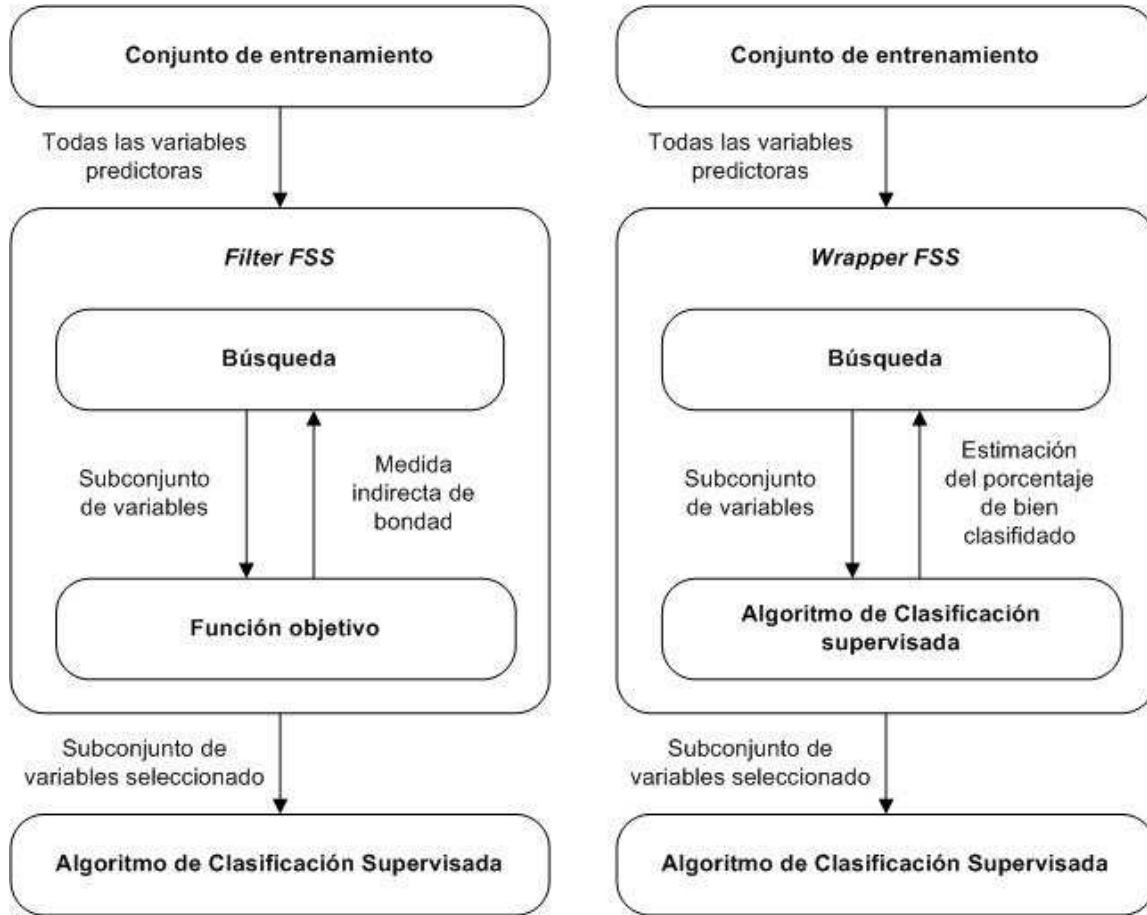
Figura 2: Diferencias entre las aproximaciones filter y wrapper a la clasificación supervisada
