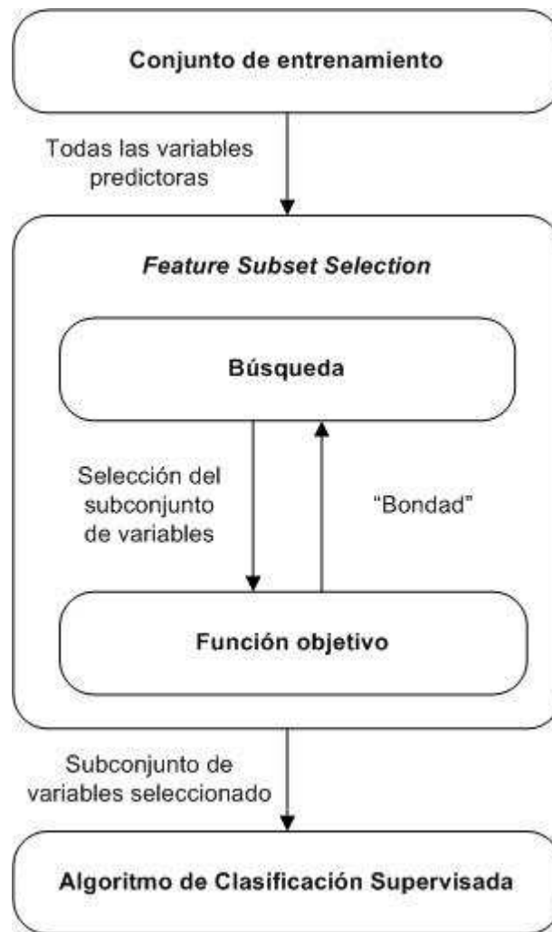
Figura 1: Esquema del procedimiento de selección de subconjuntos de variables para problemas de clasificación supervisada
