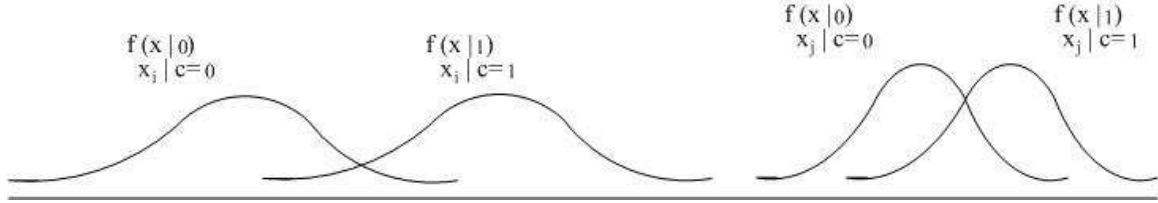
Figura 3: Funciones de densidad de las variables X_i y X_j condicionadas a los dos valores de la variable clase, C .
