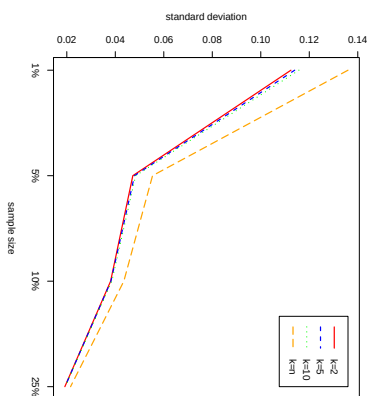
(d) C=5
